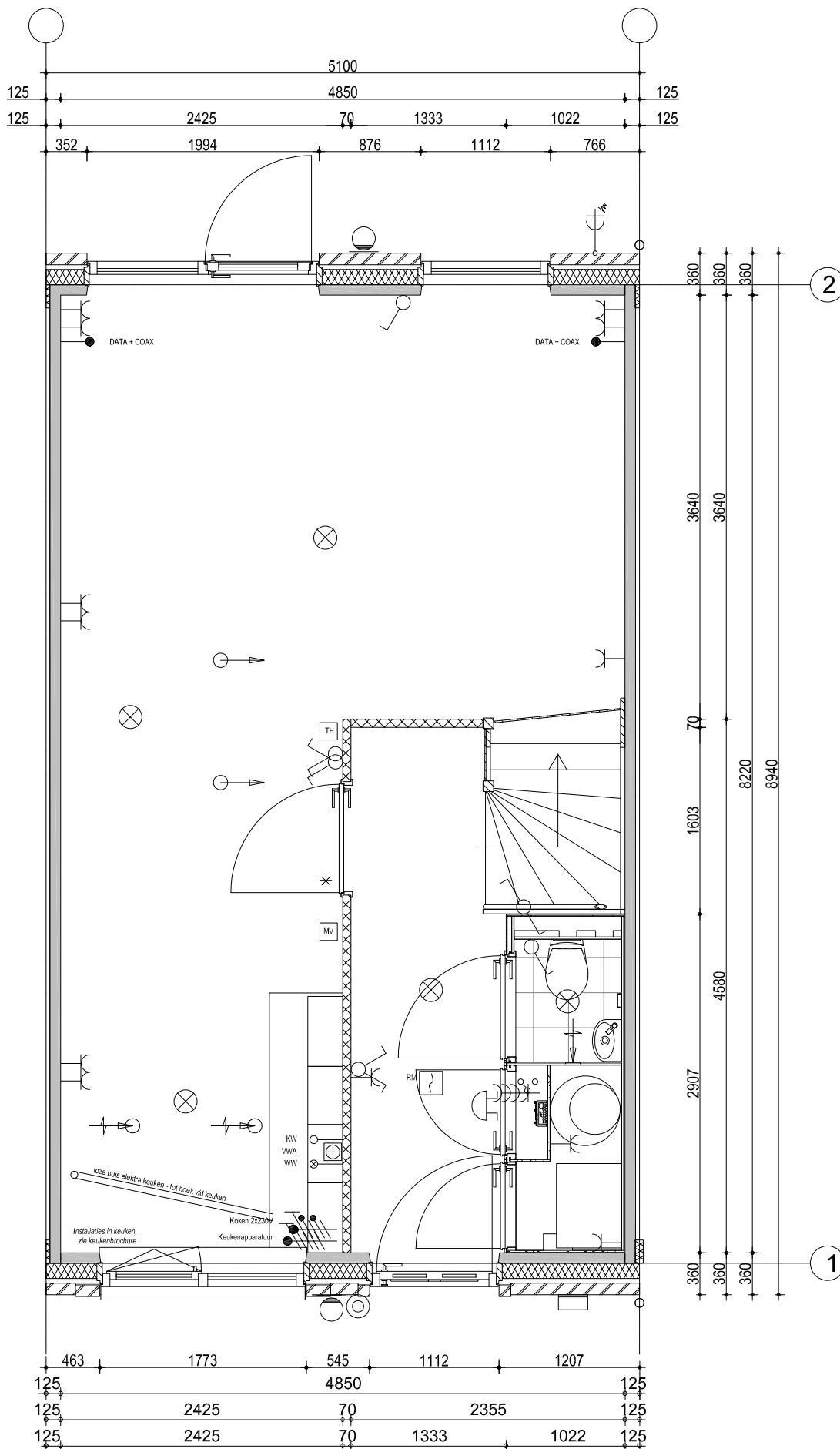
Begane grond
